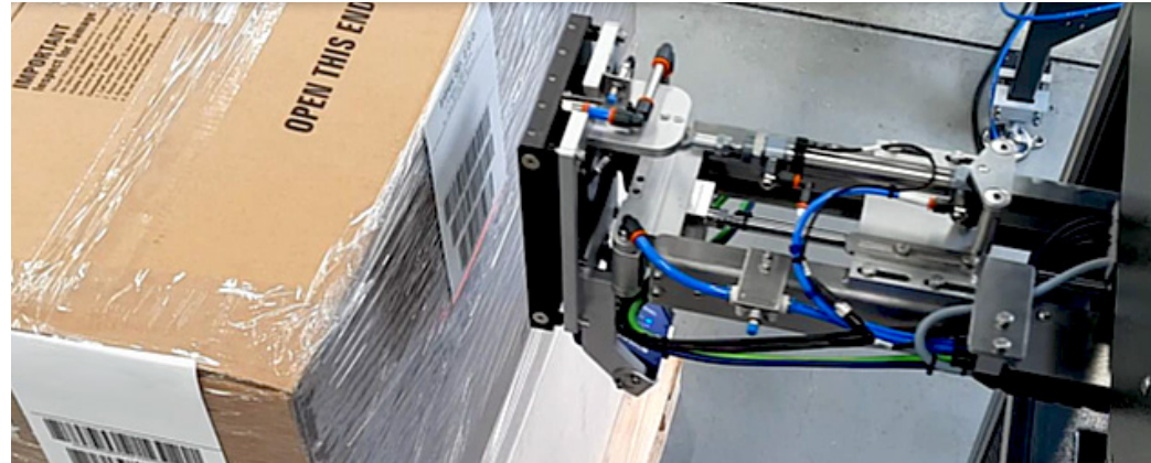
System automatyzujący aplikację etykiet logistycznych Polska
